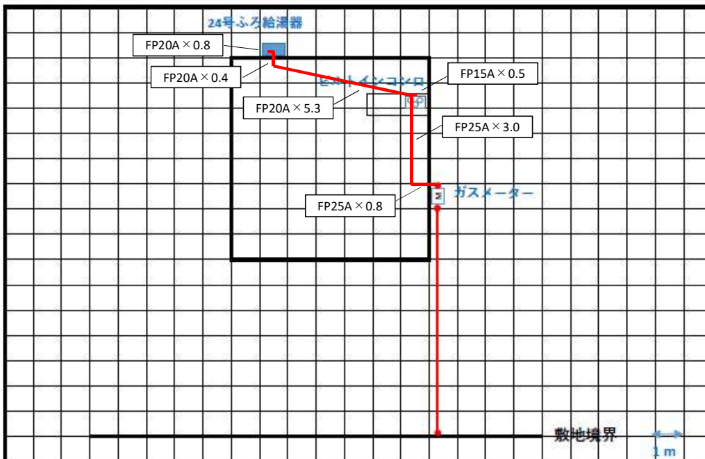
内管工事見積用平面図
